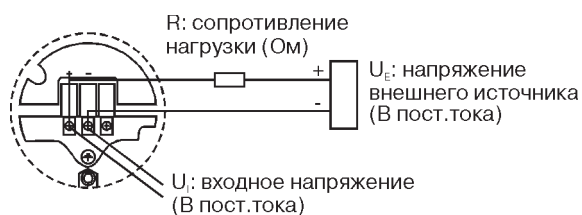
Рис. 19. Сигнал 4-20 мА/HART.
