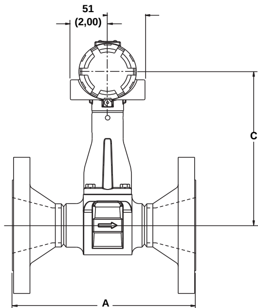
Расходомер без опции МТА
