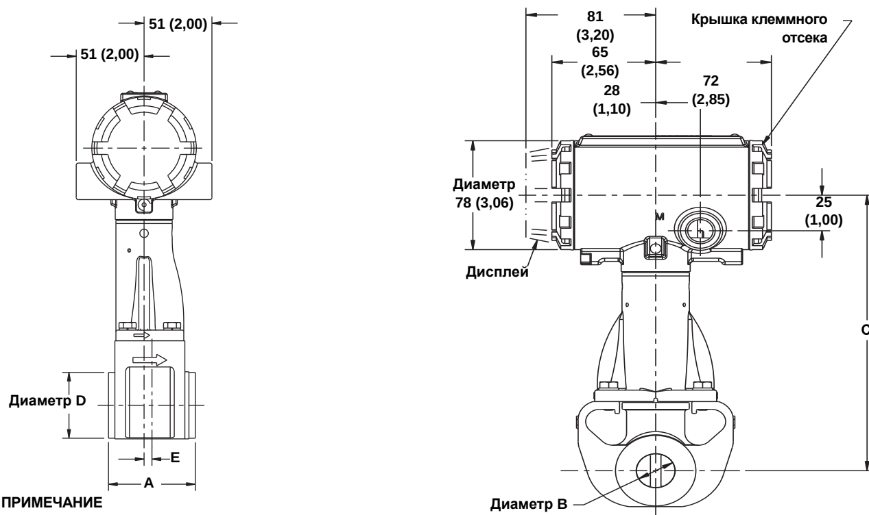
Рис. 4. Габаритные чертежи бесфланцевых расходомеров (для условных проходов 15 - 200 мм 1/2 - 8 дюймов)
