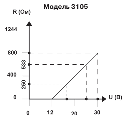
Рис. 11. Диаграммы сопротивлений для уровнемера, сертифицированного на искробезопасность.
